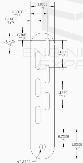
1 1 4" LONG CLIP N.T.S. FLATTENED
